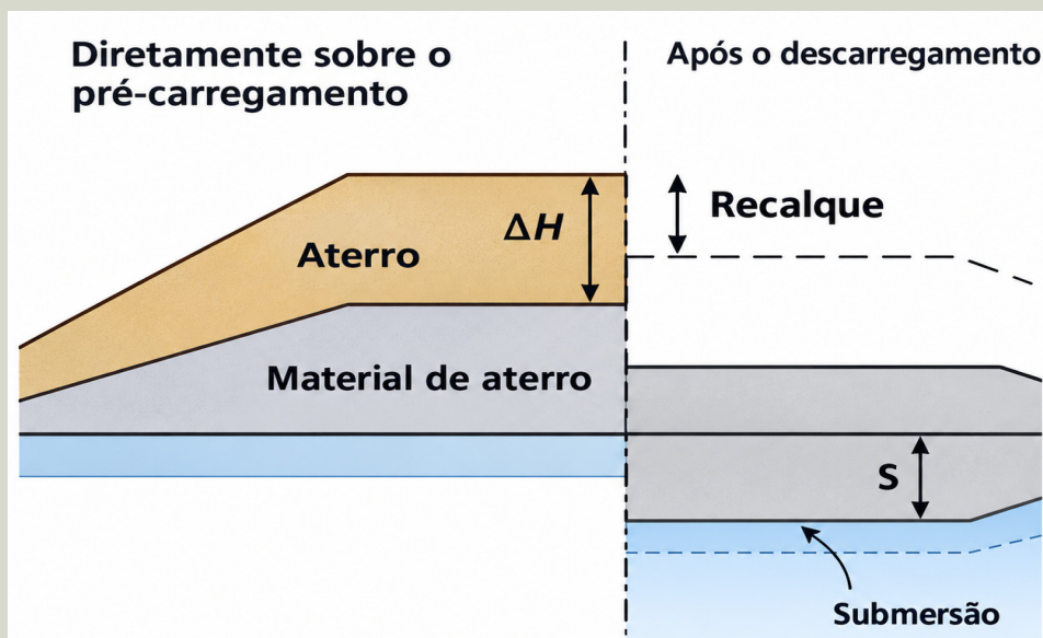
Figura 3 — Representação esquemática do aterro durante o pré-carregamento e após sua remoção, evidenciando o recalque e a alteração da geometria decorrentes do adensamento do solo mole.
