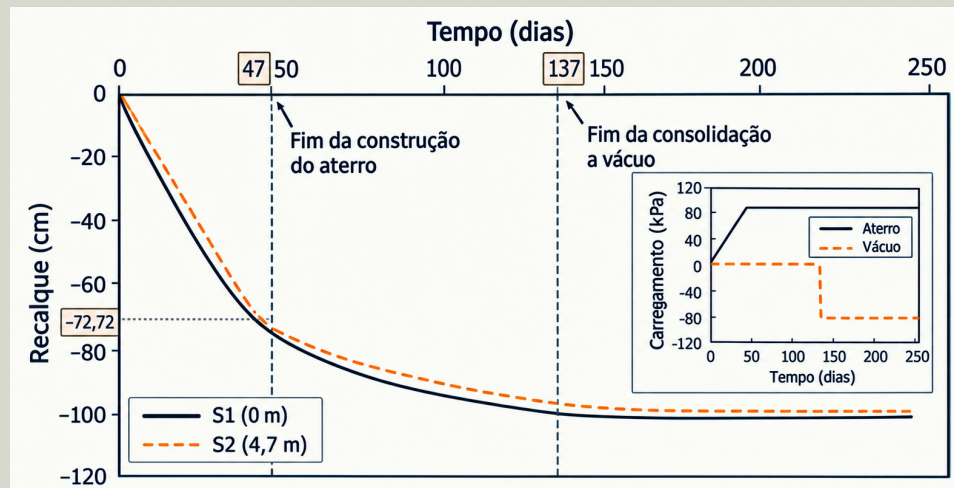
Fig. 6 - Consolidação a vácuo. Evolução dos recalques em função do tempo durante o pré-carregamento associado à consolidação a vácuo. As curvas S1 e S2 mostram o desenvolvimento dos recalques até o término da construção do aterro (47 dias) e durante a aplicação do vácuo, mantida até aproximadamente 137 dias. O gráfico inserido apresenta o histórico de carregamento do aterro e da pressão de vácuo.
