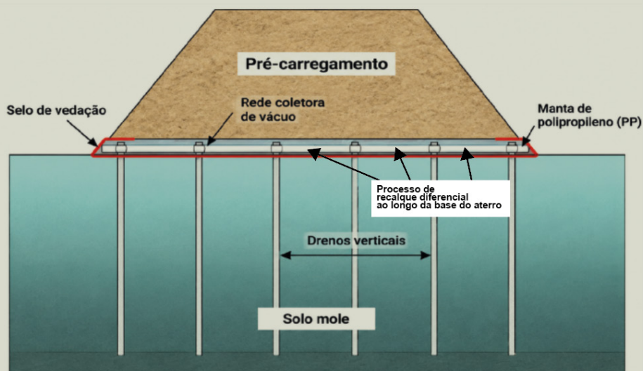
Figura 7 - Esquema típico de pré-carregamento à vácuo, mostrando o aterro, o selo de vedação, a rede coletora de vácuo, a manta de polipropileno (PP) e os drenos verticais instalados no solo mole.
