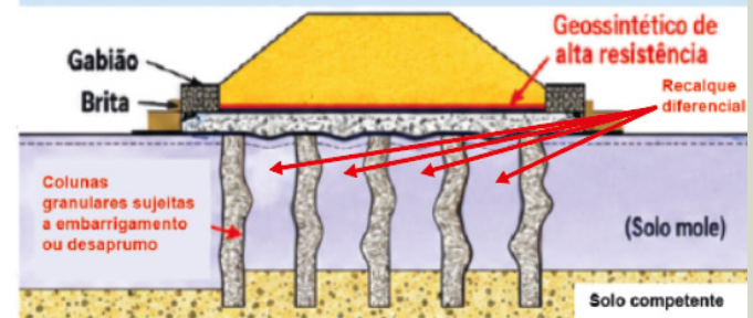
Figura 7 — Problemas de deformação em aterros sobre solos moles e soluções alternativas ou paliativas, combinando colunas de brita e geossintético de alta resistência, visando apenas atenuar recalques e deslocamentos laterais.
