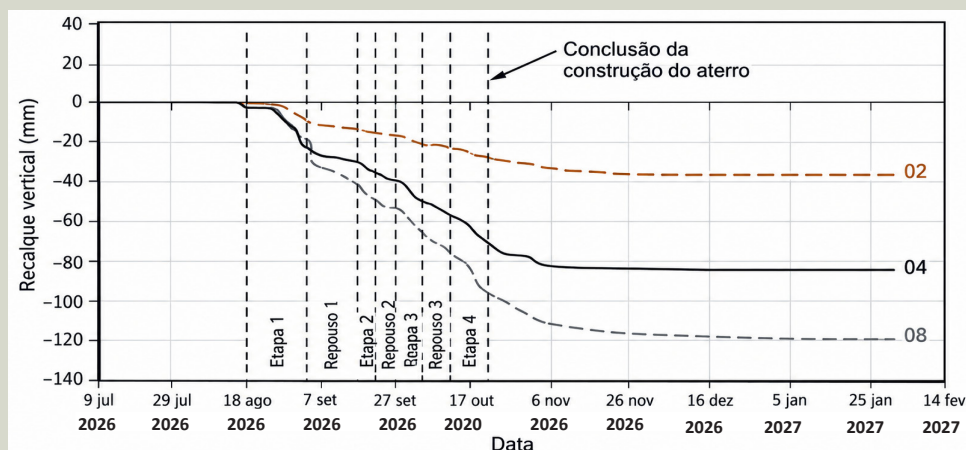
Figura 5 - Construção convencional em etapas. Evolução do recalque medido nos pontos 02, 04 e 08 durante a construção escalonada do aterro, evidenciando a resposta do solo às sucessivas etapas de carregamento e aos períodos intermediários de repouso, bem como a estabilização do recalque após a conclusão da construção.
