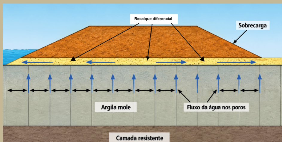
Figura 2 — Esquema do fluxo da água nos poros durante o pré-carregamento de uma camada de argila mole, evidenciando a drenagem vertical em direção à camada de areia e sua posterior dissipação lateral.
