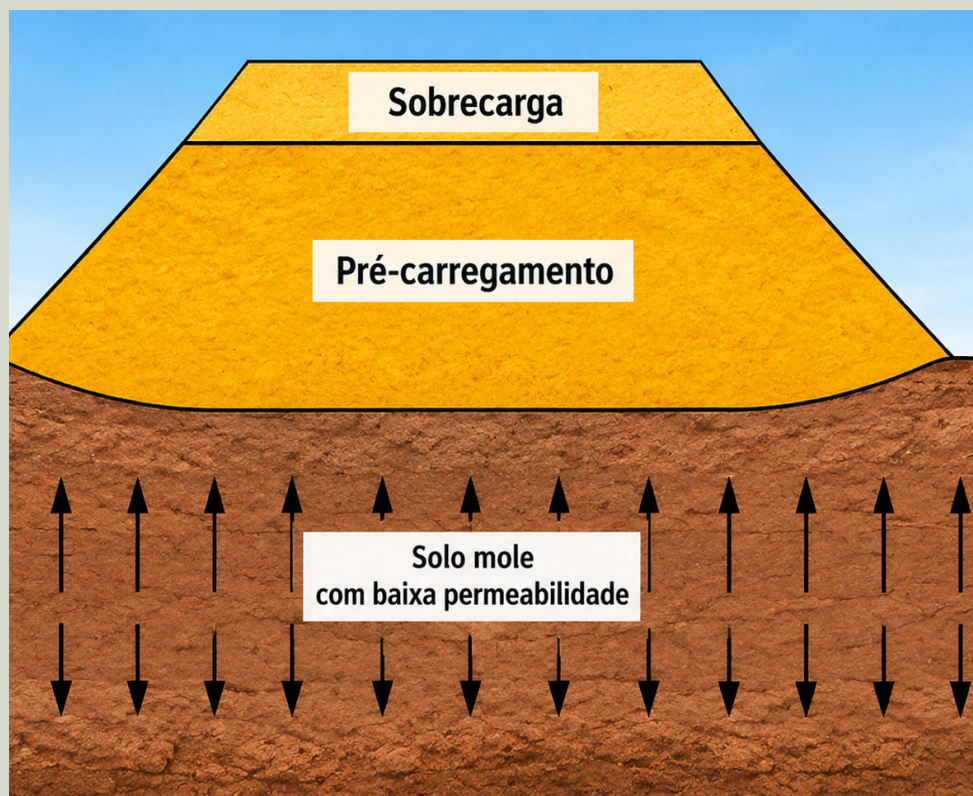
Fig. 2 - Representação esquemática do pré-carregamento em solo mole, com aplicação de sobrecarga para acelerar o adensamento e promover a dissipação das poropressões.
