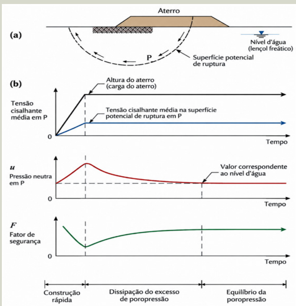
Figura 8 – Estabilidade de aterros sobre solos argilosos moles: (a) configuração geométrica do aterro e mecanismo potencial de ruptura; (b) evolução das tensões cisalhantes, das poropressões e do fator de segurança durante a construção e após sua conclusão.
