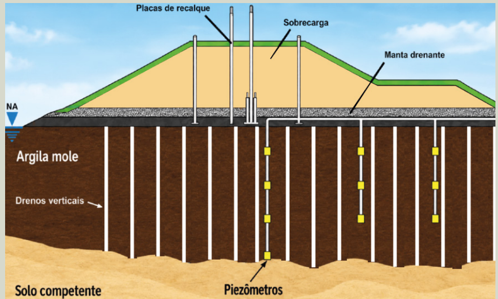
Figura 5 — Seção típica de pré-carregamento com drenos verticais, mostrando a sobrecarga, a manta drenante e a instrumentação por placas de recalque e piezômetros para acompanhamento do processo de adensamento da argila mole.
