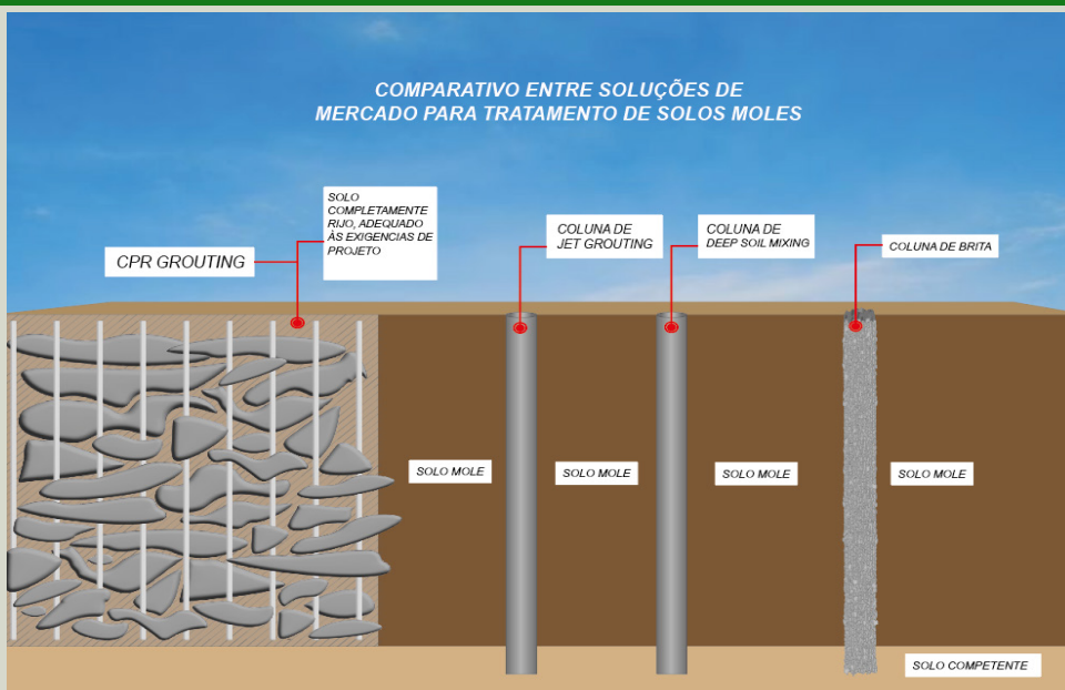
Fig. 6 – Comparação entre métodos de tratamento de solos moles para obras rodoviárias. O CPR Grouting promove o melhoramento efetivo do maciço, aumentando sua rigidez e resistência, por meio da consolidação e do geoenrijecimento da massa de solo, readequando o comportamento geotécnico do terreno eliminando recalques totais e diferenciais. Em contraste, técnicas como colunas de brita, Deep Soil Mixing e Jet Grouting atuam predominantemente como elementos estruturais verticais, promovendo a transferência parcial das cargas para camadas mais profundas ou mais resistentes, sem melhorar o solo mole entre as colunas, resultando em concentrações de tensões, movimentações diferenciais e redução da eficiência em solos muito moles, heterogêneos ou espessos. Nestas condições, a eficiência destas técnicas costuma ser limitada, frequentemente não ultrapassando 50%.
